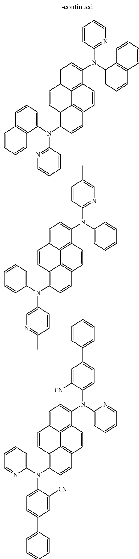
FD2
