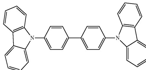
CDBP
